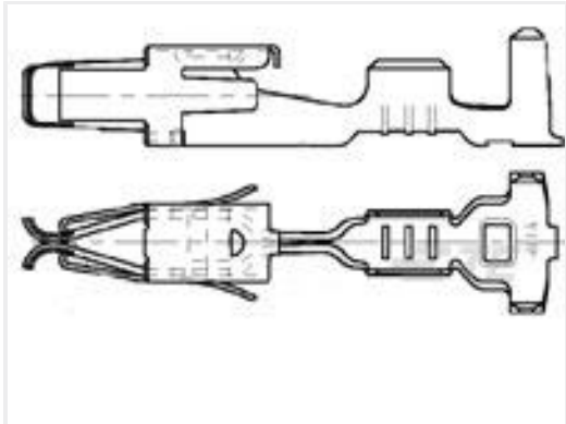
TE 产品编号185026-1 JPT F REC 2.8 Contact SWS Sn
