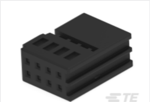
TE 产品编号1418789-1 8POS MQS REC
