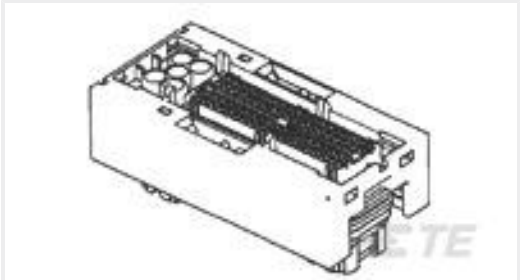
TE 产品编号CAT-M8793-T273 MQS, 母端和公端
