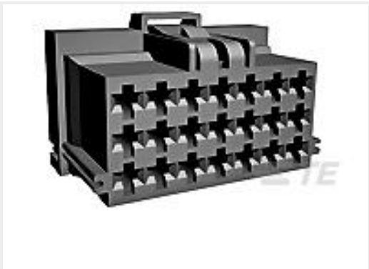
TE 产品编号8-968975-1 MCP2.8 GEH 21P
