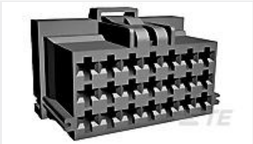
TE 产品编号8-968975-1 MCP2.8 GEH 21P
