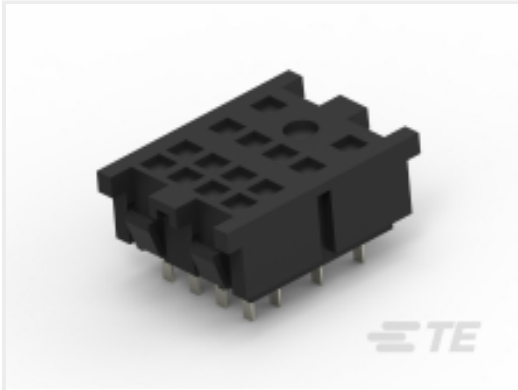
TE 产品编号1419106-3 27E023=SOCKET,KH,14,PCB,PHEN,BL
