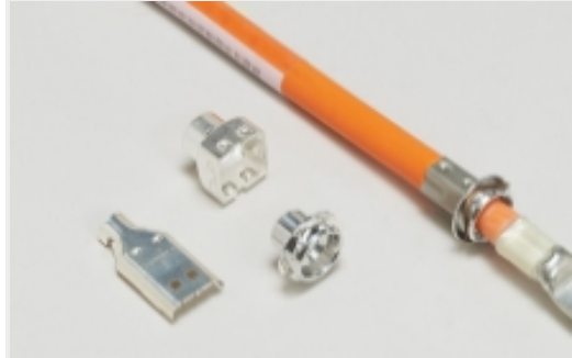
汽车连接器 EMC 屏蔽(3)
