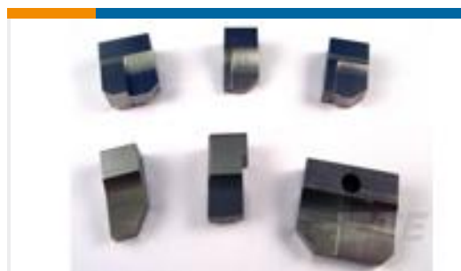
TE Part #1338686-3 ANVIL
