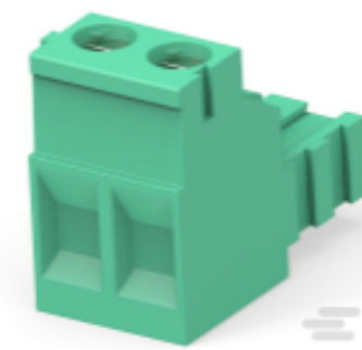
TE Part # 282805-2 TERMI-BLOK PLUG STACKING 2POS.
