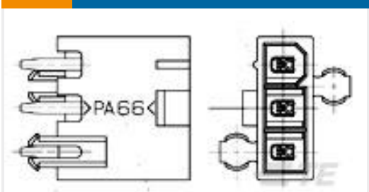
TE Part #2029054-3 3P VAL-U-LOK SR HDR SN V2 W/DH
