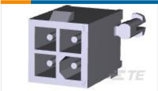
TE Part #770874-1 04P MINI UMNL HDR ASSY SN
