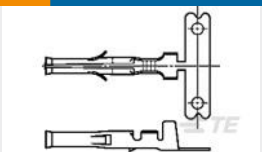
TE Part #350628-2 .062 COMM P&S SOK PTPPHBZ
