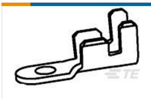
TE Part #40990-1 WELD TAB TAB 20-16 AWG TPSTL
