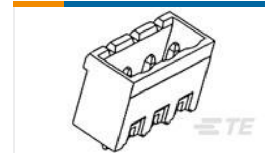
TE Part #796980-4 4 POS TERMI-BLOK VERT HDR 7.62
