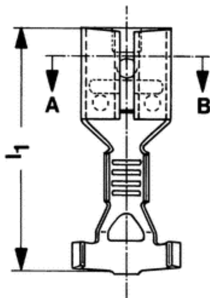
Schnitt A - B
