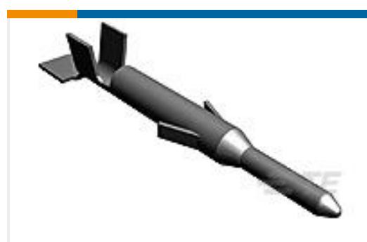
TE Part #1586537-1 MINI UMNL PIN SN 16 AWG
