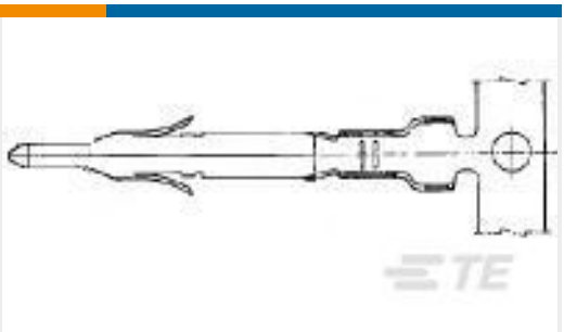
TE Part #170363-1 MINI UNIVERSAL M-N-L PIN LP
