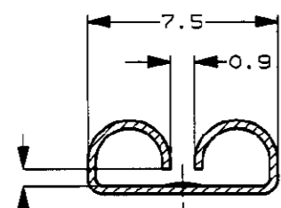
SECT. 断面 A-A
