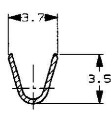
SECT. 断面 A-A
