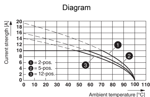
Type: MSTB 2,5/...-STF-5,08 with MDSTBV 2,5/...-GF-5,08
