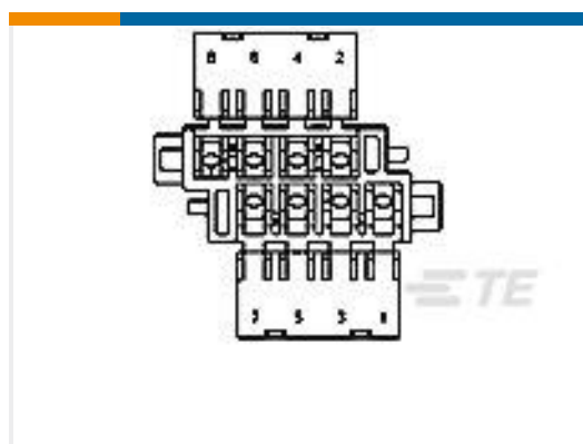
TE Part #365063-3 8P TAB HSG BLK
